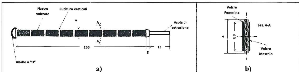
Figura 1 Vista frontale della fascia in configurazione aperta (a) e sezione della stessa (b). Disegno non in scala ed a titolo puramente esemplificativo.
